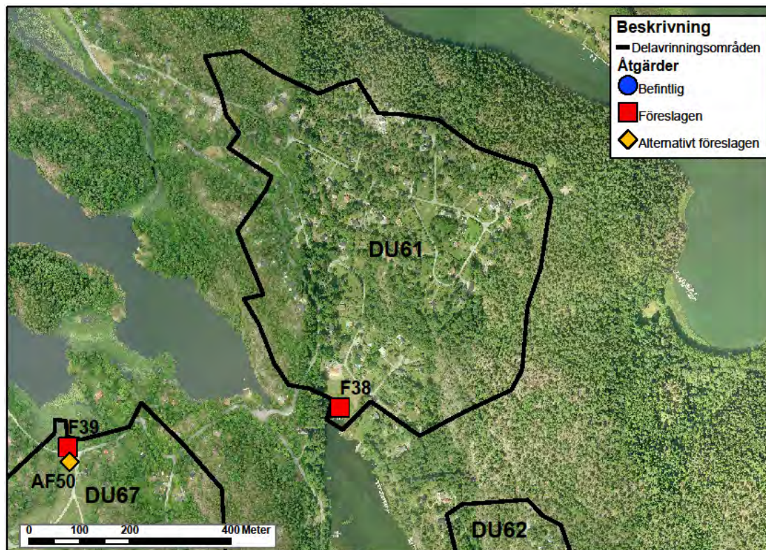
Bild 41. Inom delavrinningsområde DU61 föreslås att dikenas reningsfunktion förbättras genom breddning och/eller fyllning med makadam (F38).
