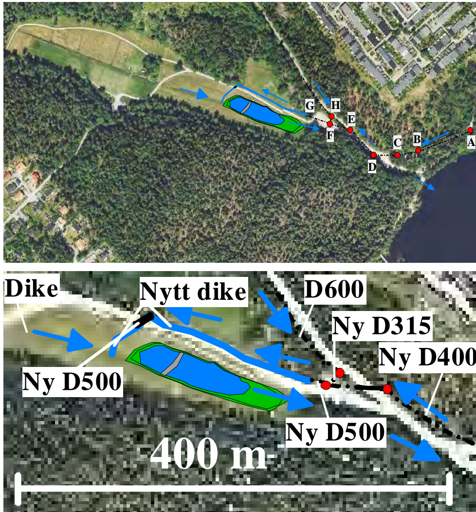
Bild 13. Skiss från förprojektering av reningsanläggning vid Prästängen. Den övre bilden visar ny ledningssträckning där A-H markerar olika ledningssträckor och den nedre bilden utgör en mer detaljerad skiss på ledningarna och diken vid anläggningen.
